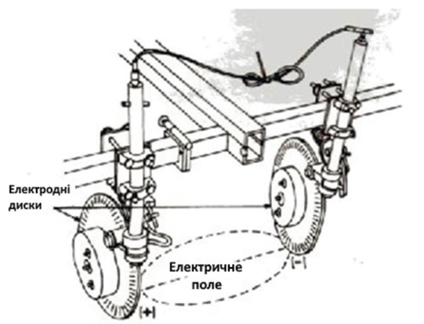
Рисунок 2 – Схема технологічного процесу роботи Soil Doctor [Freddy A. et al, 2021]
